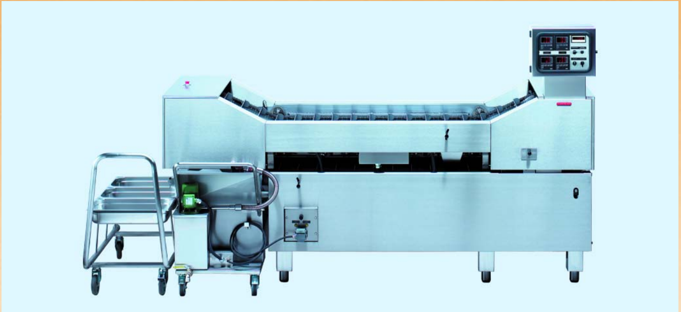
EBA 100 mit Ölfilterwagen und Transportwagen für GN-Behälter / with an oil filter trolley and a transport trolley for GN containers / avec chariot de filtration de l'huile et chariot de transport pour les récipients gastronome
